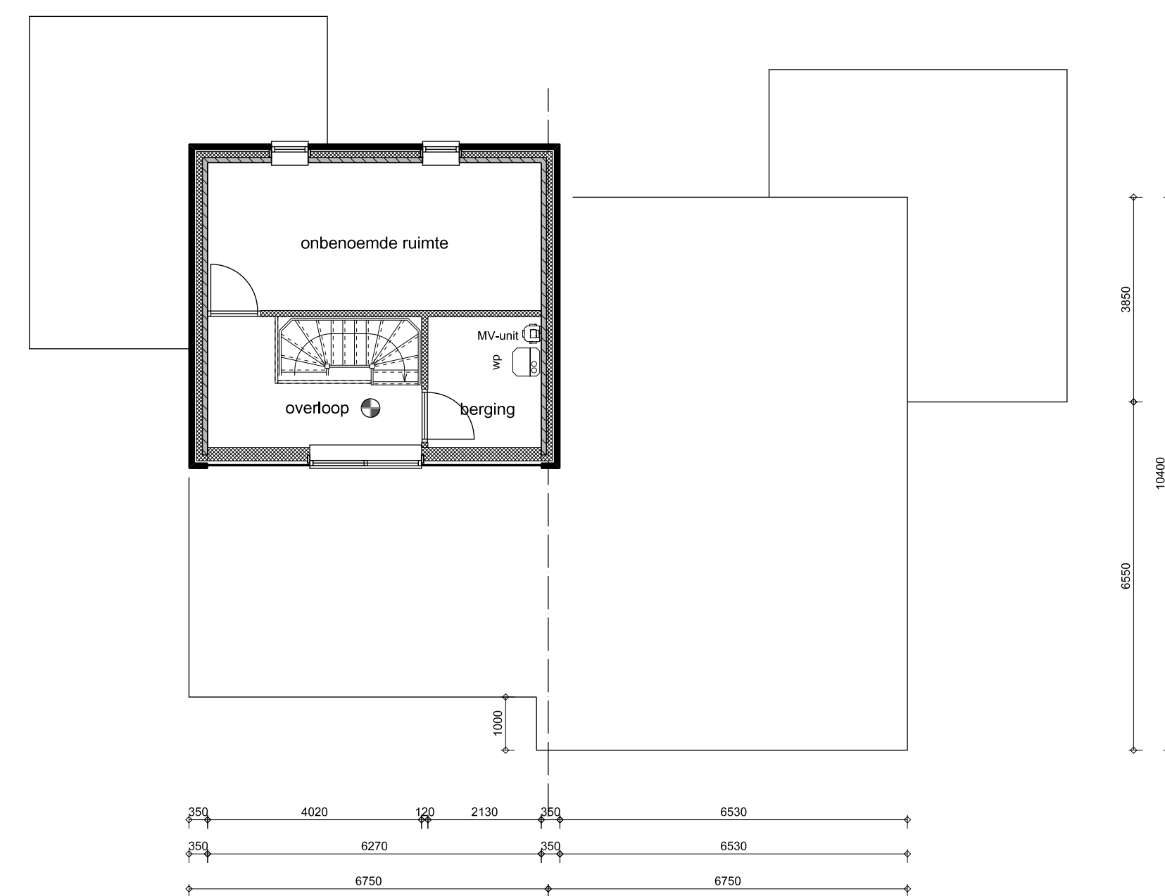
VERDIEPING 2
